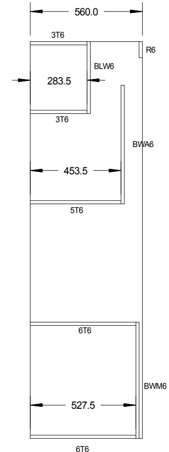
End Elevation
